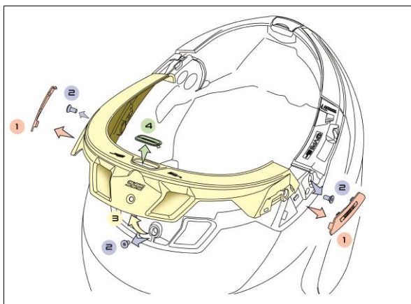
Fig. 4C – SOLO PARA EL CASCO N100-6, N120-1
